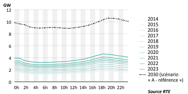
Courbes journalières moyennes au pas horaire de la production éolienne corrigée, de 2014 à 2023 et en projection pour 2030 (scénario « A-référence » du Bilan Prévisionnel)
