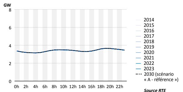
Courbes journalières moyennes au pas horaire de la production hydraulique au fil de l'eau corrigée, de 2014 à 2023 et en projection pour 2030 (scénario « A-référence » du Bilan Prévisionnel)
