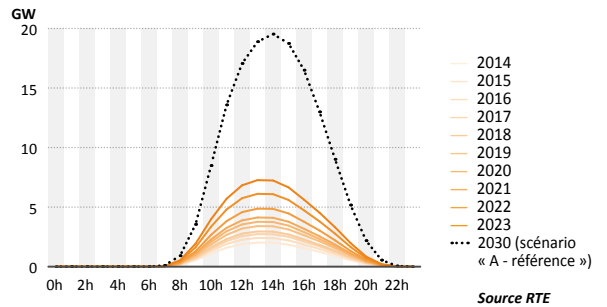
Courbes journalières moyennes au pas horaire de la production solaire photovoltaïque corrigée, de 2014 à 2023 et en projection pour 2030 (scénario « A-référence » du Bilan Prévisionnel)
