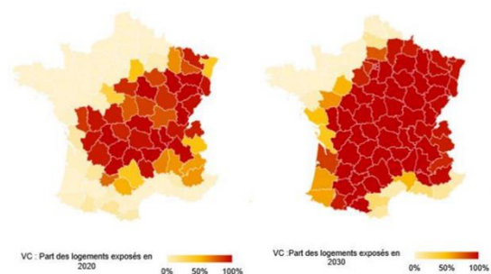
Figure 11 : Part des logements exposés à au moins 20 jours de vagues de chaleur par an par département
