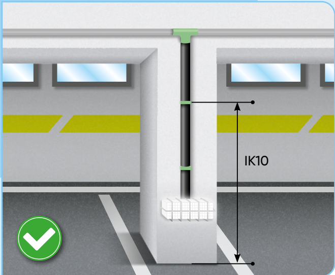
Résistance mécanique dans les parcs de stationnement. Exemple : parking de plus de 100 m 2
