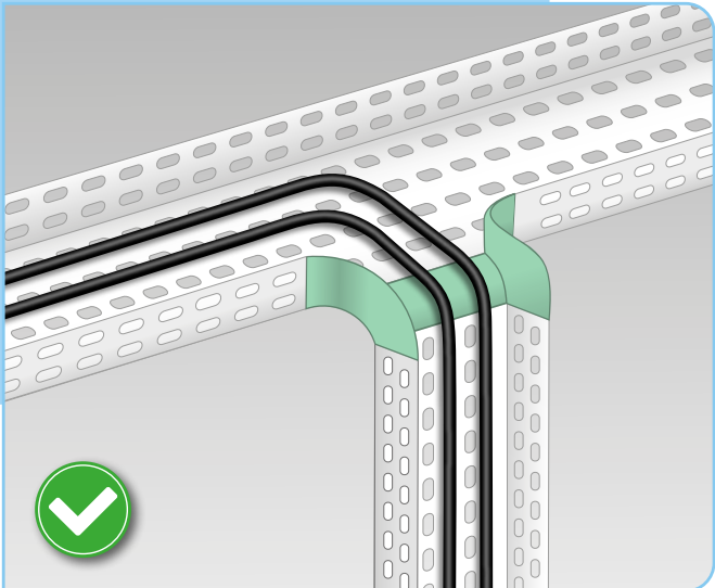
Protection des câbles et des utilisateurs
