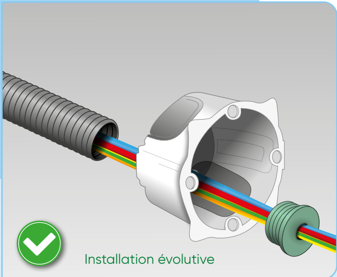
Garantie d'étanchéité à l'air conformément à la Réglementation Thermique
