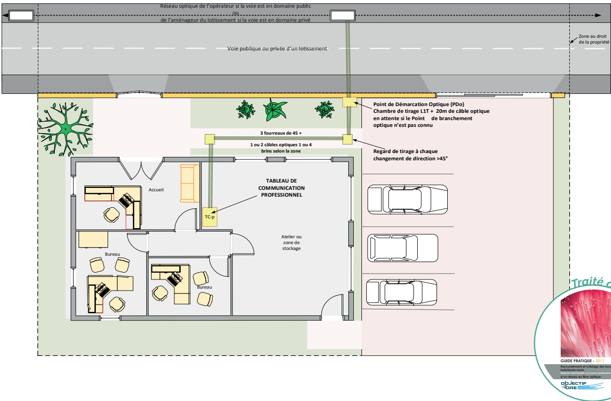
Fig 76 : Raccordement d'un local individuel
