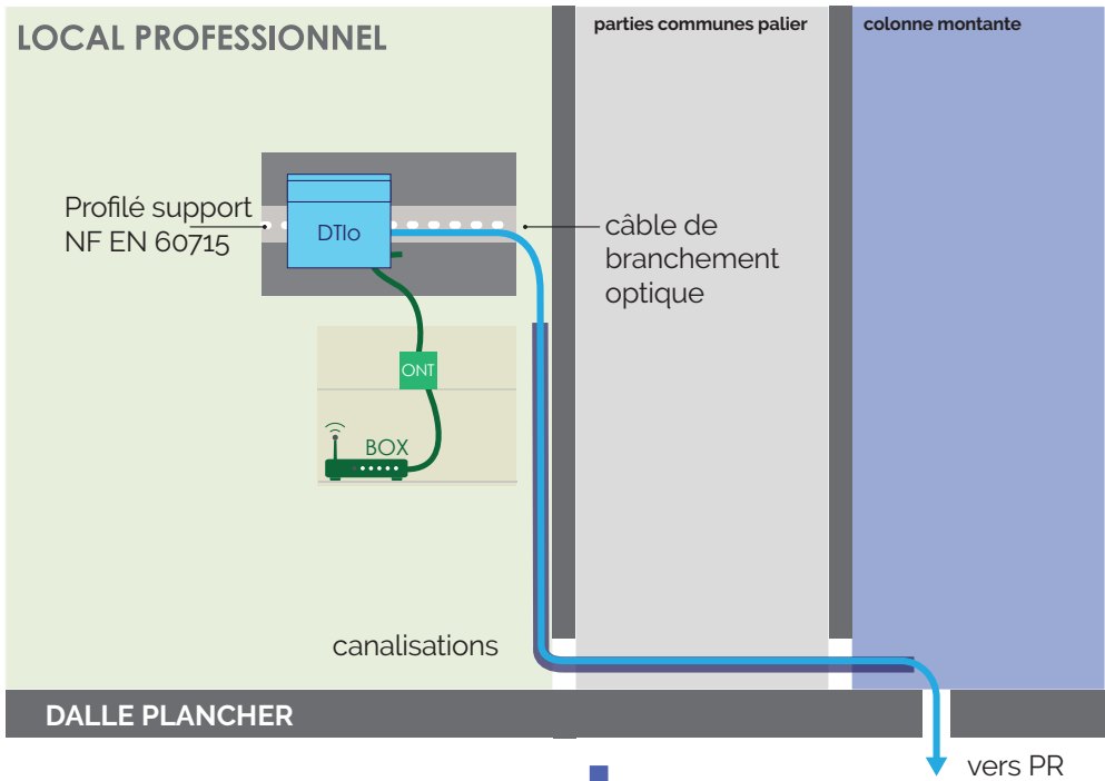
Fig 35 : Installation type sans PBO
