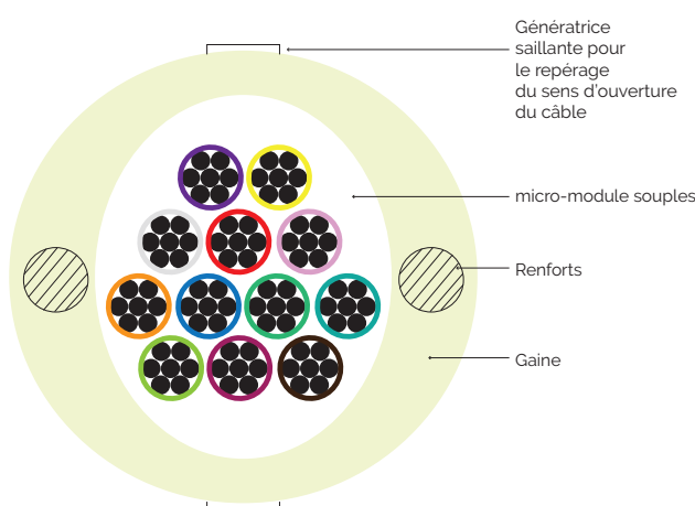
Fig 64 : La capacité en fibres peut aller jusqu'à 144Fo préconnectorisées
