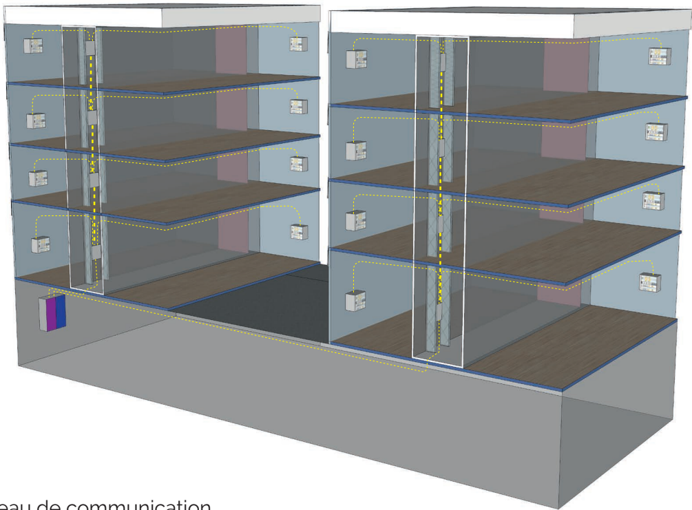
Fig 52 Immeuble de bureaux avec 2 bâtiments
