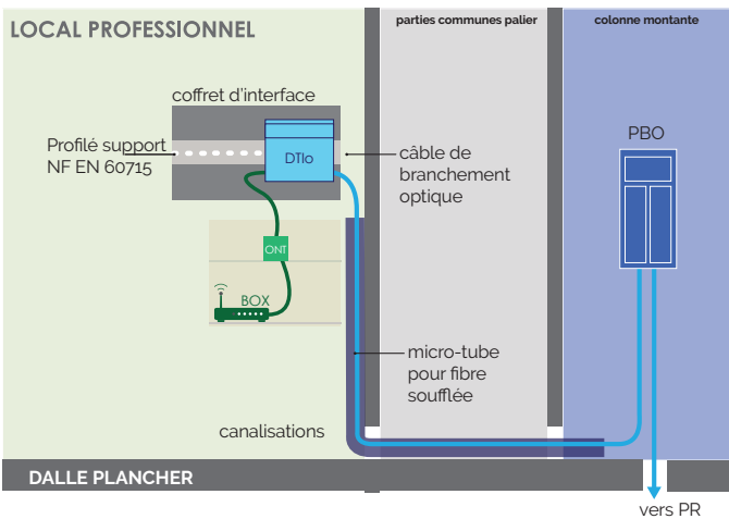
Raccordement par Fibre en micro-tube soufflée
