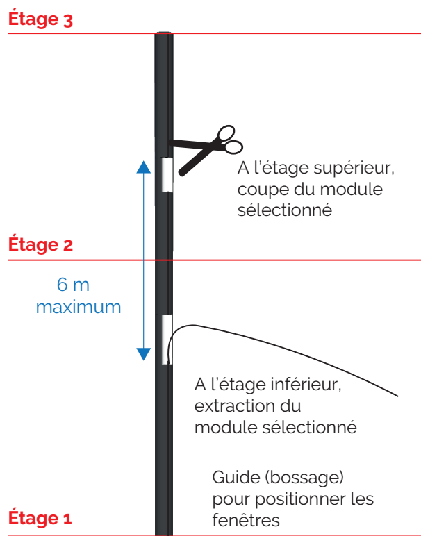
Fig 54 : Extraction de modules
