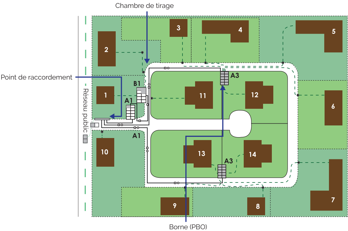
Fig 90 : Diagramme de câblage pour un campus privé
