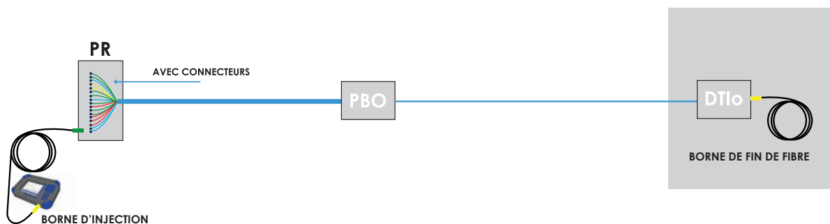
Fig 81 : Test d'un liaison PR/DTIo par réflectométrie
