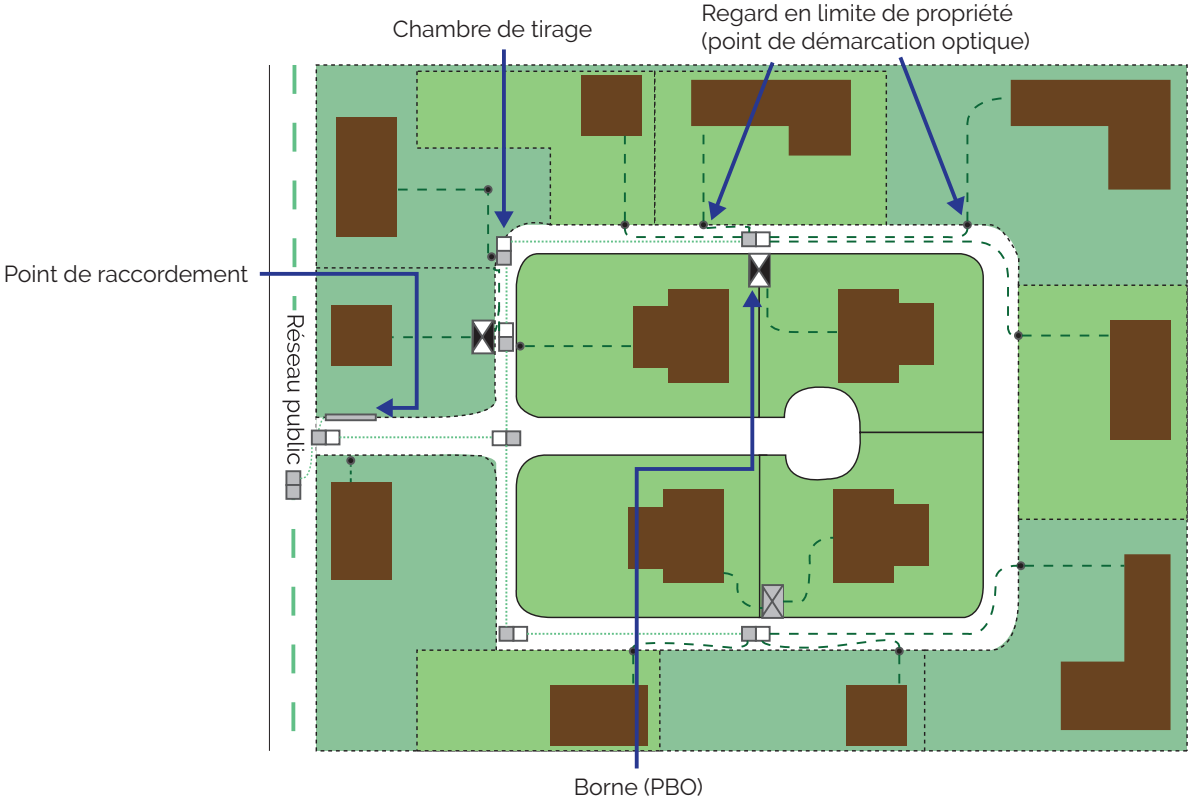
Fig 89 : Plan de VRD (cheminement pour les campus privés)
