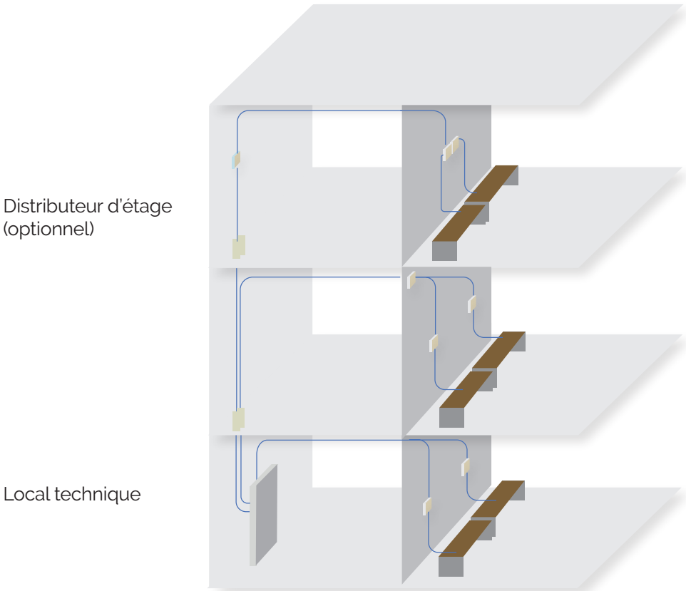
Fig 77 : Exemple d'organisation du réseau local d'entreprise
