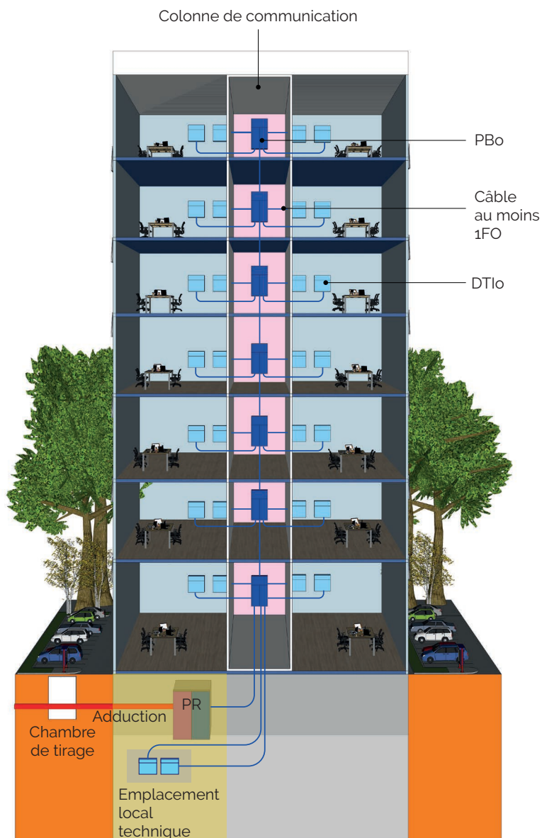
Fig 8 : Cas des immeubles nécessitant une architecture réseau avec PBo : \geq 12 accès
