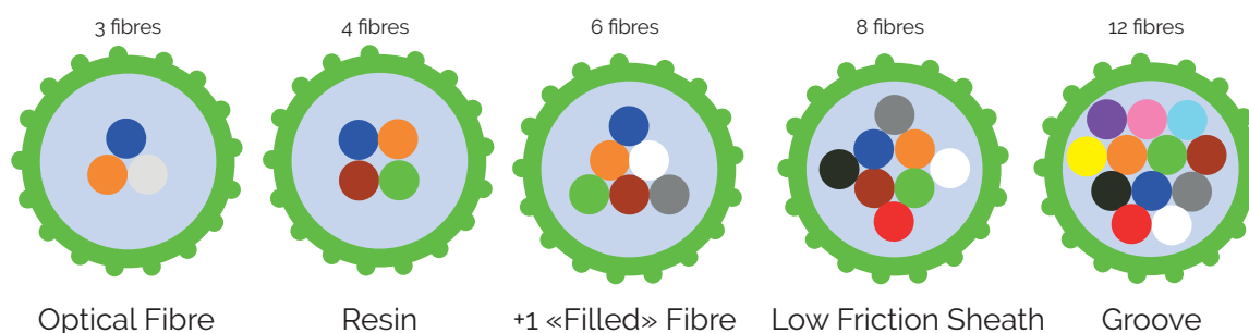
Fig 58 : modules soufflables
