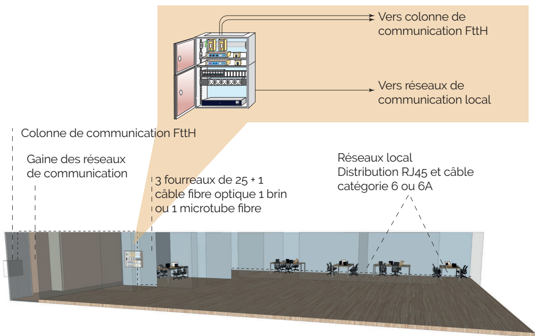
Fig 78 : Exemple de distribution dans un local profession avec un coffret de communication professionnel étendu
