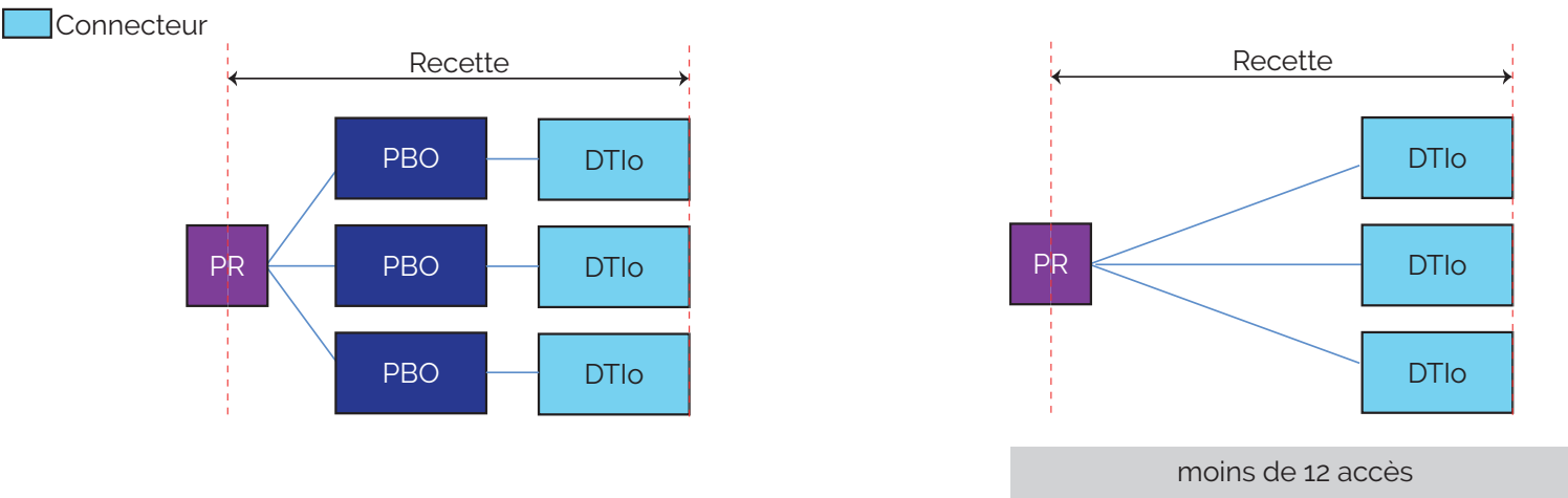
Fig 82 : Centre commercial / Pépinière d'entreprise
